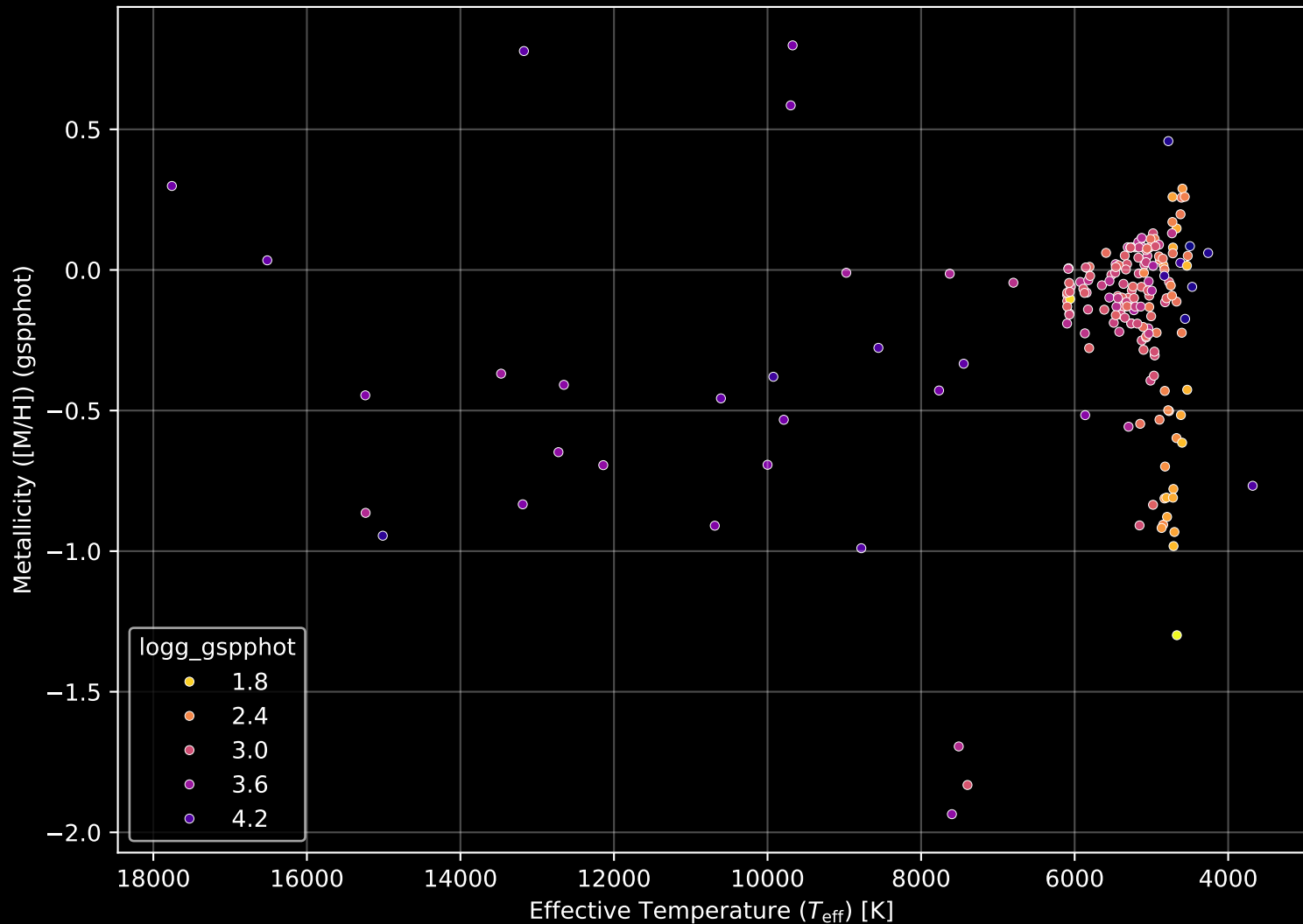
APOGEE DR17 Field: [173-04] Stellar Population Parameters (n= 192)
